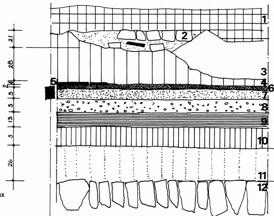
croquis de la coupe stratigraphique
